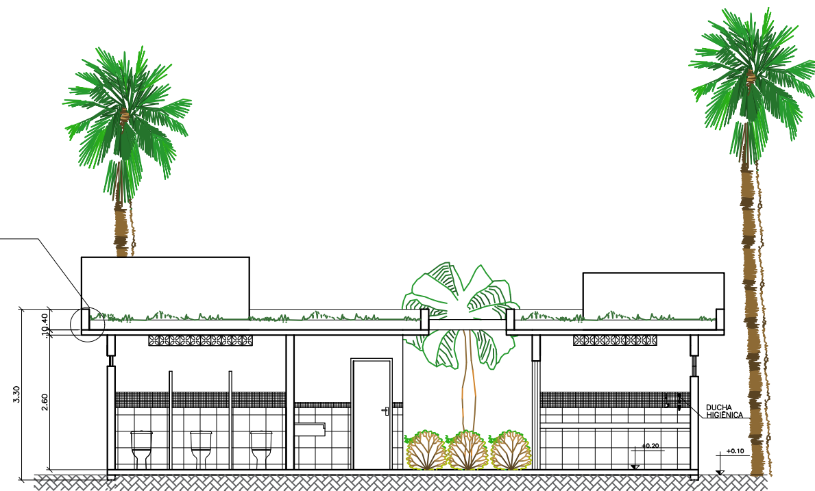
1 CORTE 1 ESCALA 1/100
