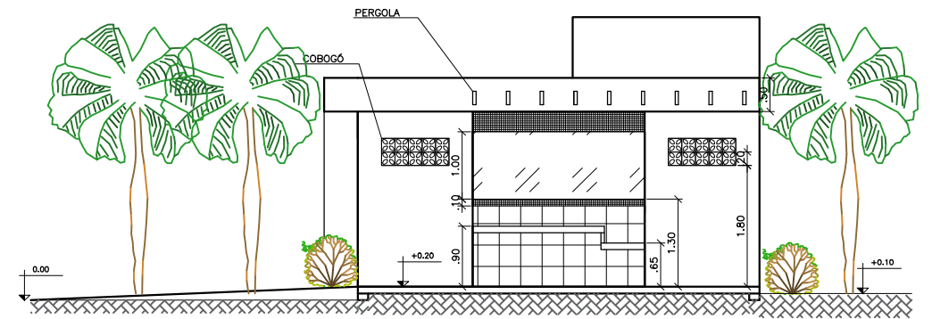
3 CORTE 3 ESCALA 1/100
