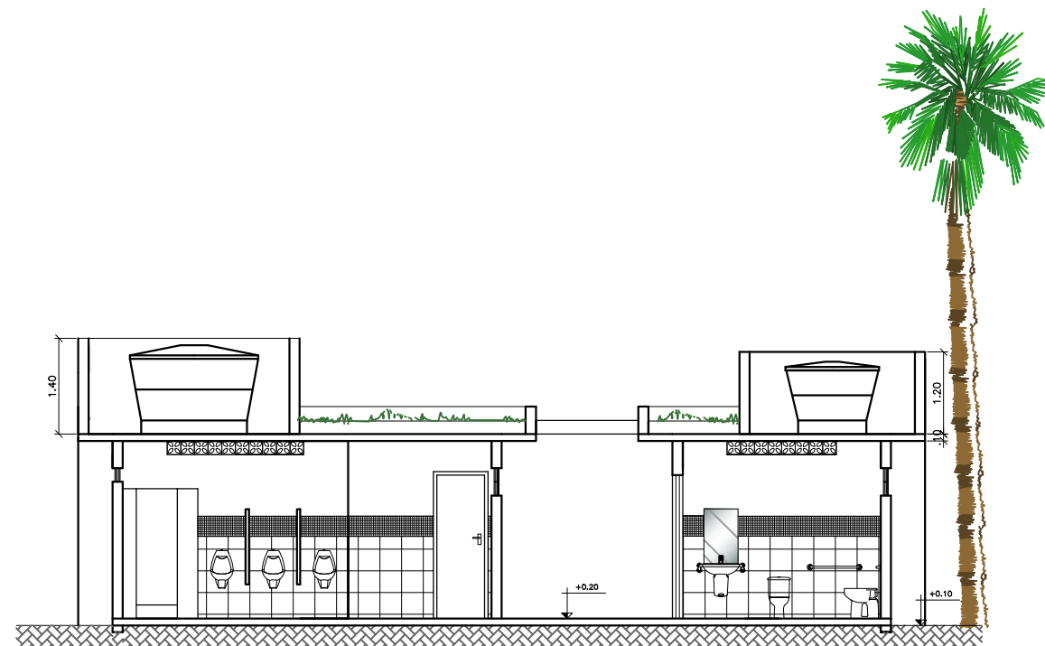
2 CORTE 2 ESCALA 1/100
